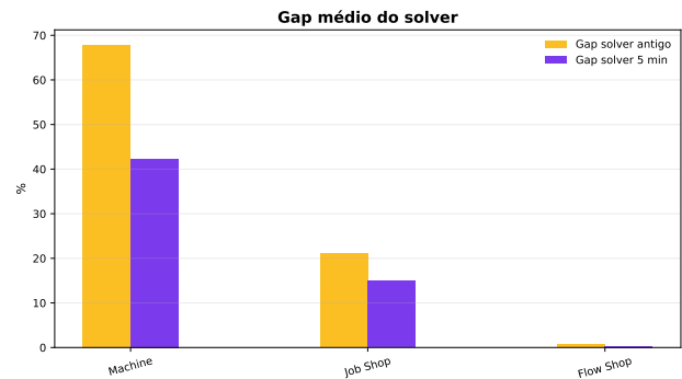
Figura 4: Gap solver médio por problema
