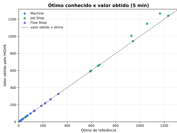
Figura 6: Ótimo conhecido versus valor obtido
