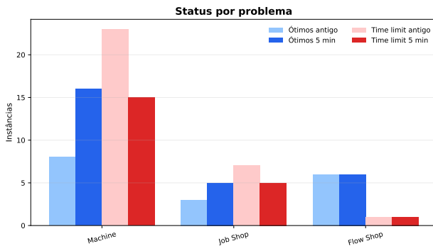
Figura 1: Status por problema
