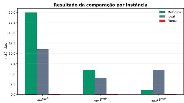
Figura 2: Resultado da comparação por problema
