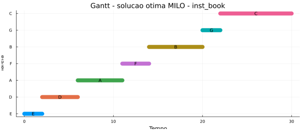
Figura 10: Machine Scheduling - instância inst_book
