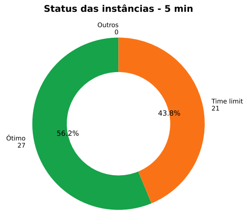
Figura 9: Status na execução de 5 minutos
