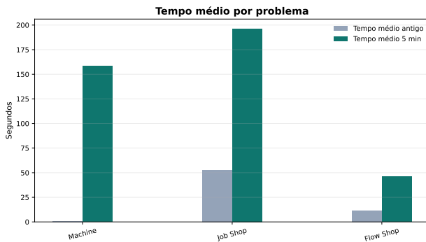
Figura 3: Tempo médio por problema
