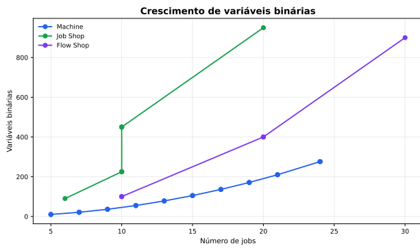
Figura 8: Variáveis binárias por tamanho
