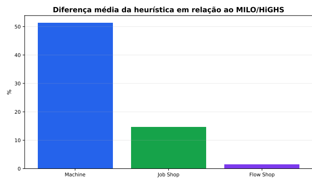
Figura 7: Heurística versus MILO/HiGHS
