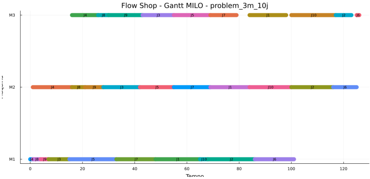
Figura 12: Flow Shop Scheduling - instância problem_3m_10j
